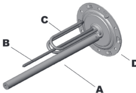
Figure 1 - Résistance thermoplongée + anode en magnésium
