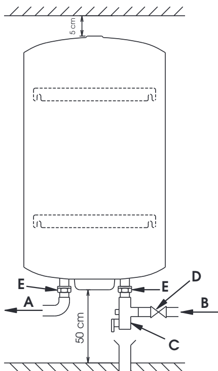
Figure 6 - Cotes d'installation
