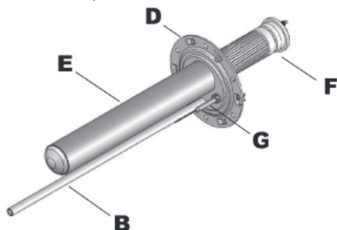
Figure 3 - Résistance stéatite + anode PROfessional TECH
