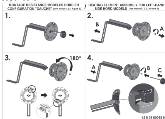
Figure 8 – Montage résistance modèles HORD en configuration "gauche"
