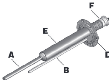
Figure 2 - Résistance stéatite + anode en magnésium
